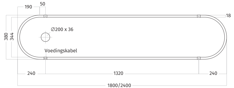
bovenaanzicht
